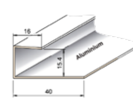
Abschlussprofil Aluminium 8236
