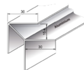
Außenkantenprofil Aluminium 8234
